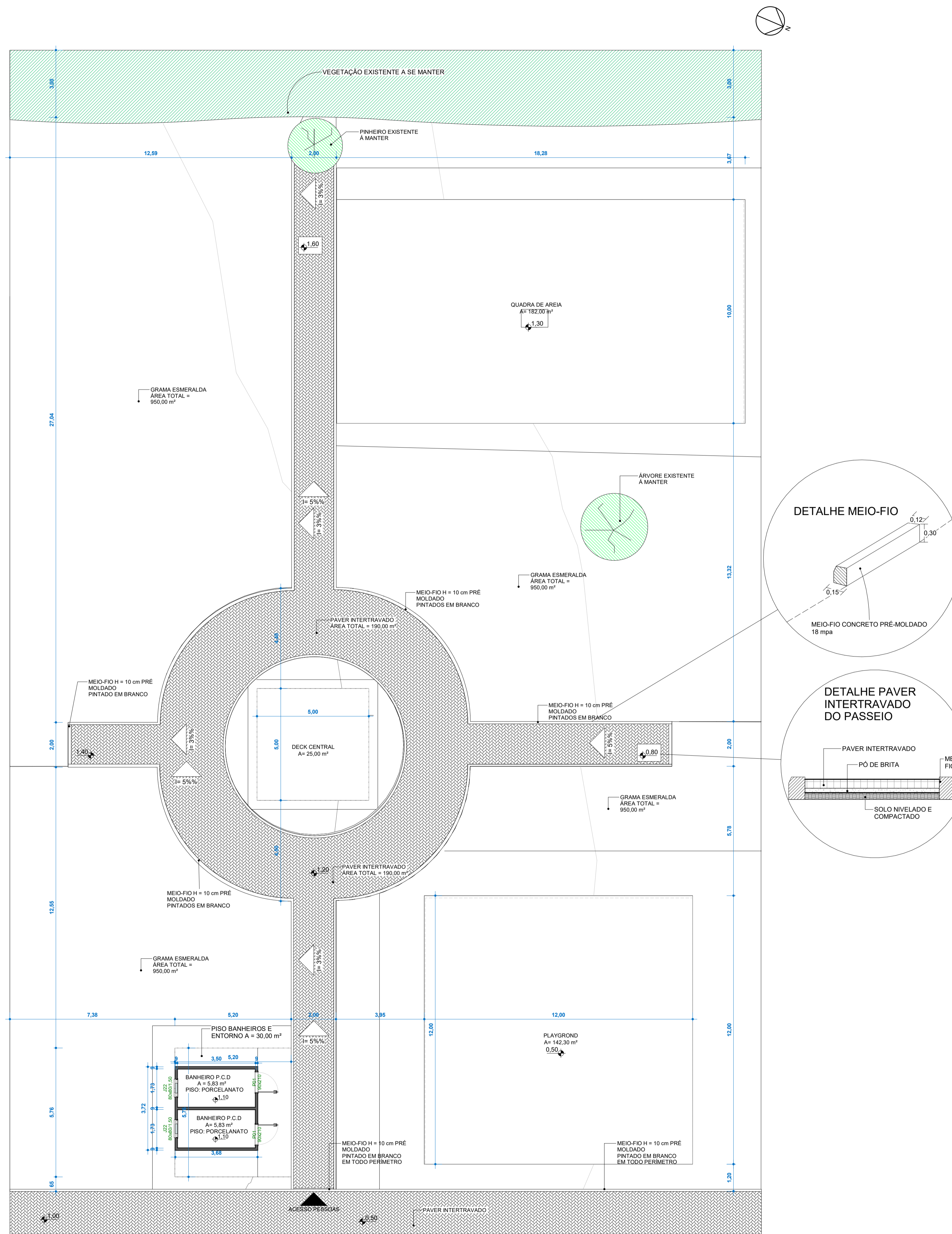
1 Planta Baixa Geral 1 : 100
