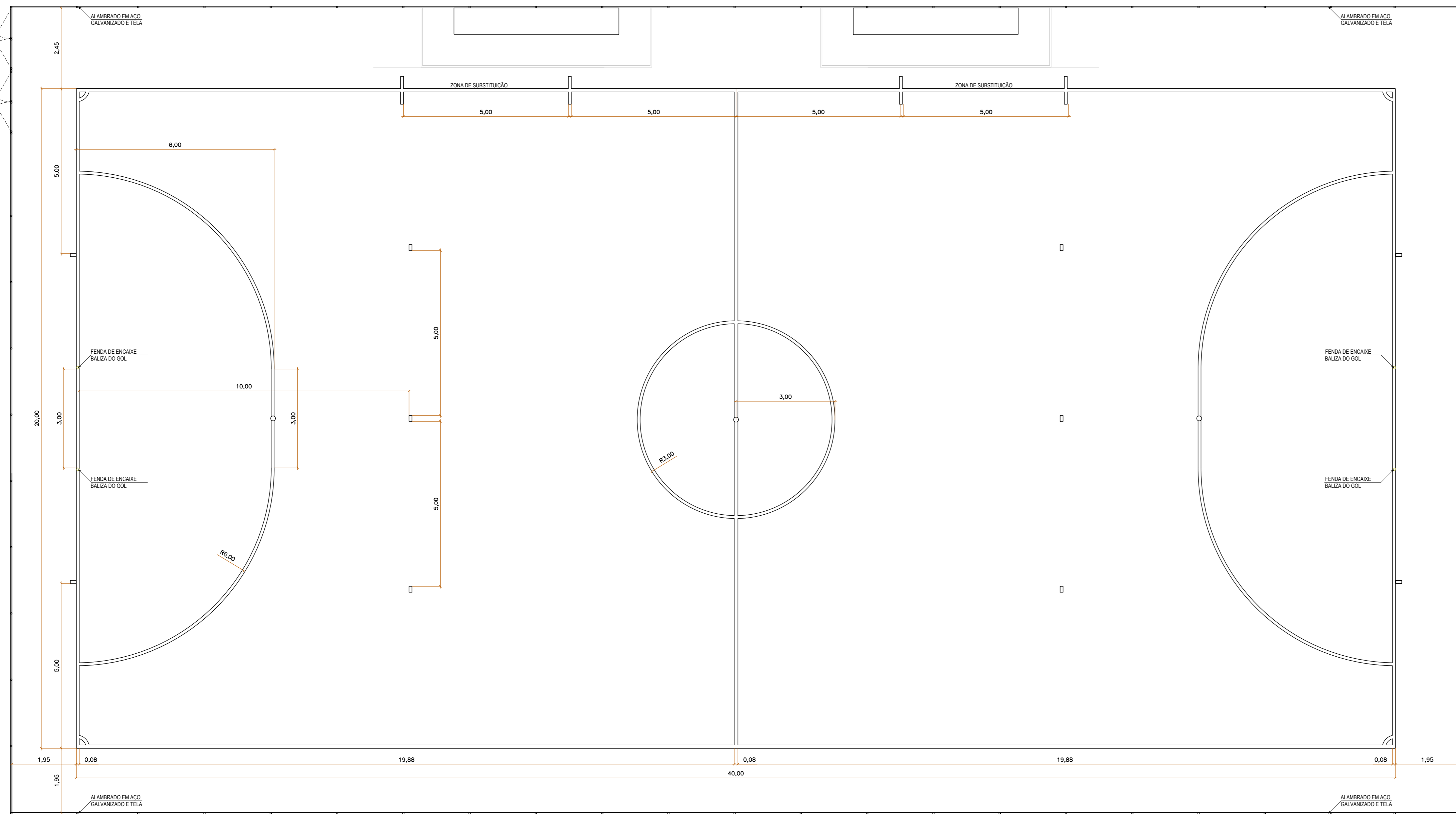
QUADRA ESPORTIVA - QUADRA DE FUTSAL ESCALA 1/75
