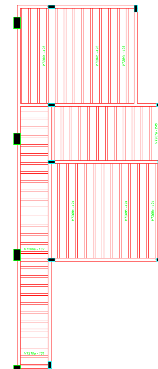
Planta de vigotas pré-moldadas escala 1:50
