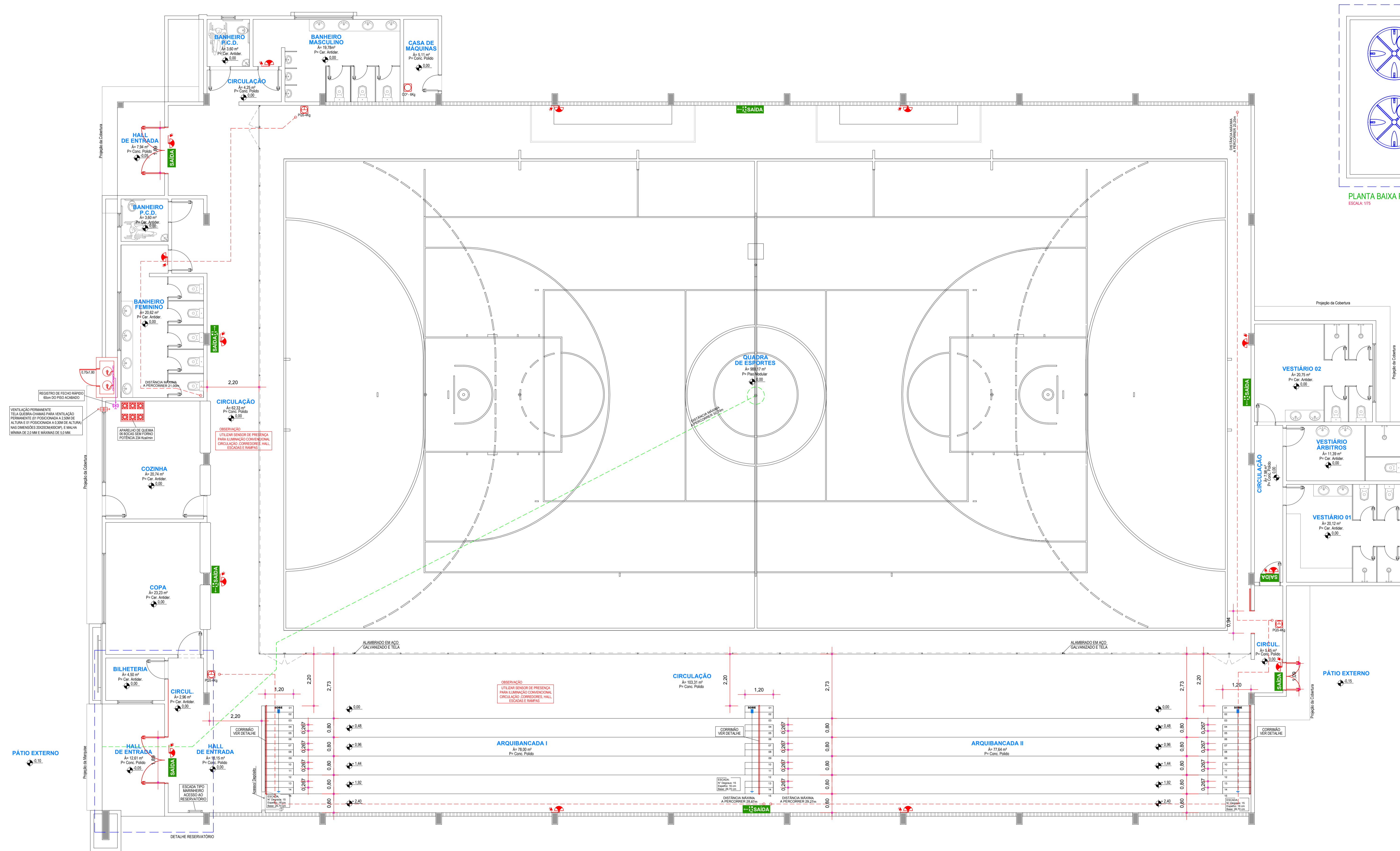
PLANTA BAIXA PAVIMENTO TERREO ESCALA: 1/15
